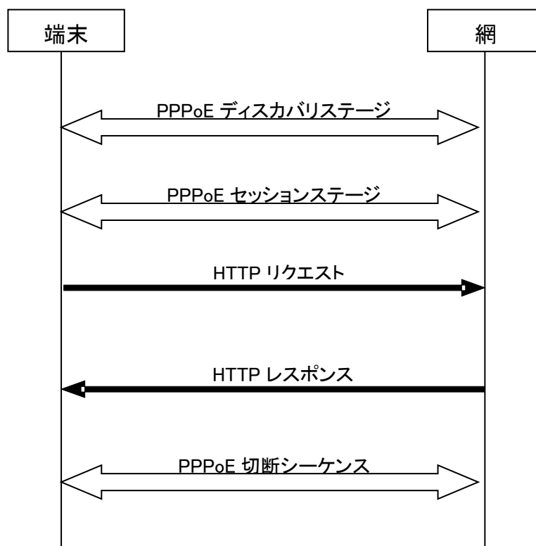
図 2.A1-1 端末自動設定シーケンス例（「B フレッツ」に対応する端末の場合）
