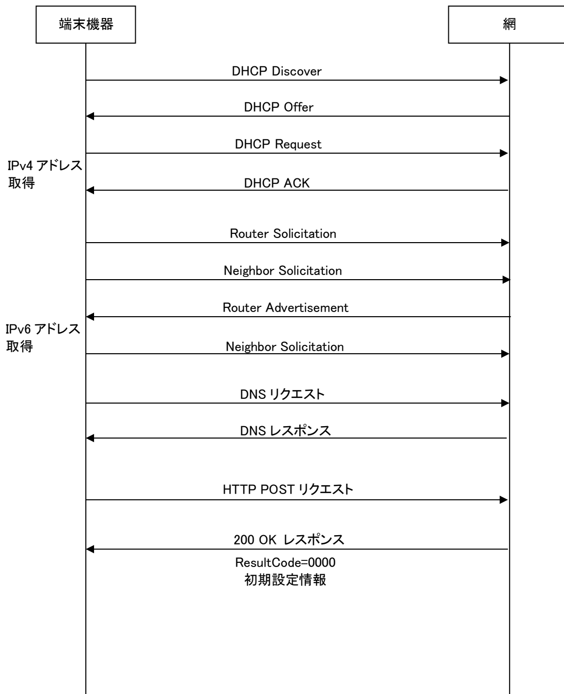
図 2.A2-1 端末自動設定シーケンス例（「フレッツ・光プレミアム （注1） 」に対応する端末の場合）
