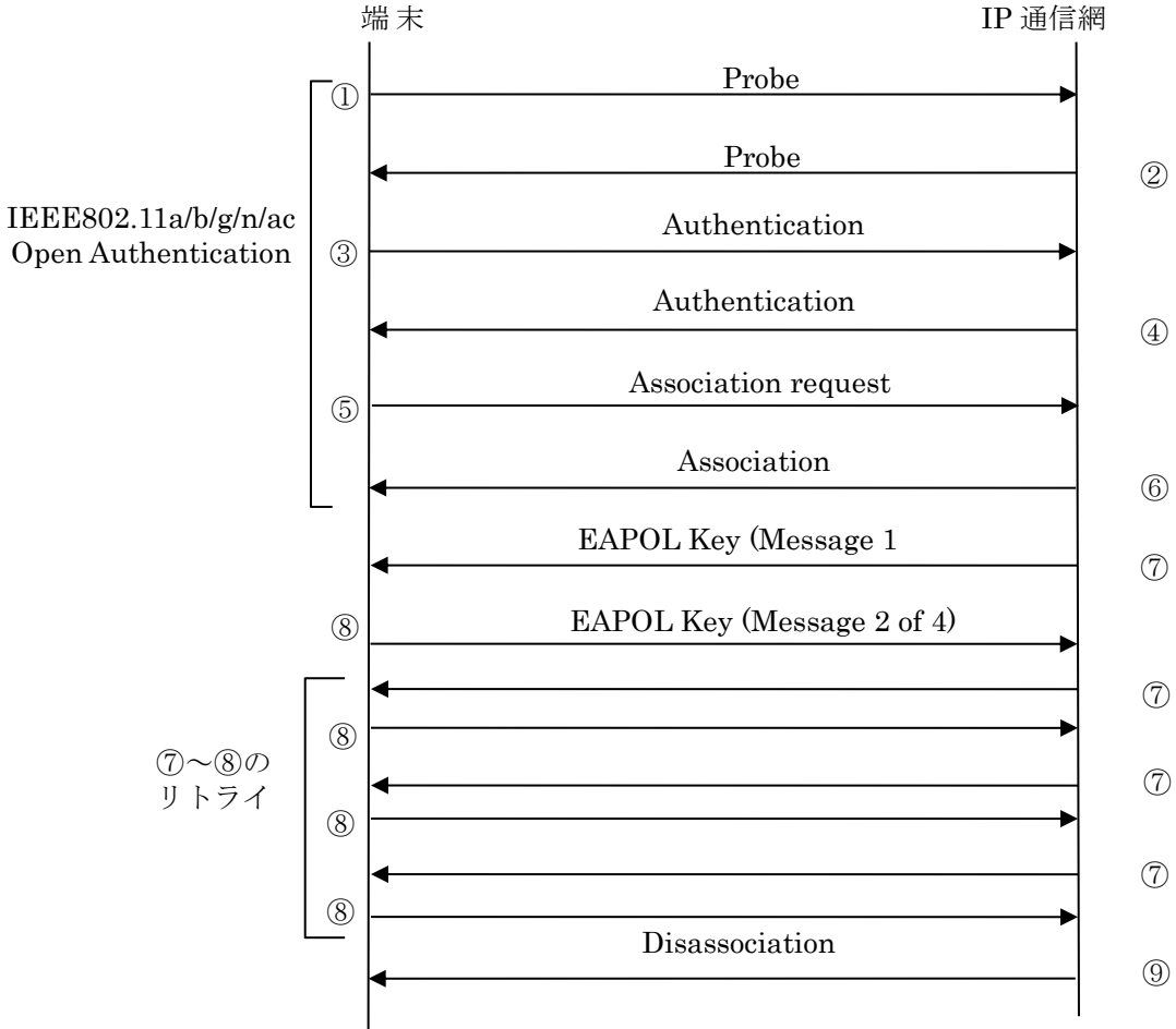
図 3.2 接続失敗シーケンス（例）
