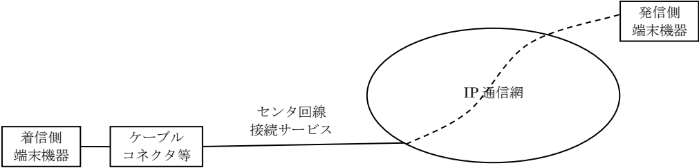
図 1.1 本サービスの基本構成
