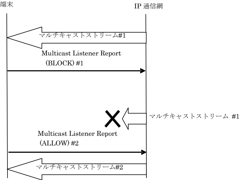
図 4.3 チャンネル切り替えシーケンス例
