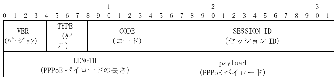
図 6.2 Ethernet ペイロードフィールドのフォーマット
